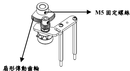
【扇形傳動齒輪】
