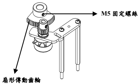
【扇形傳動齒輪】
