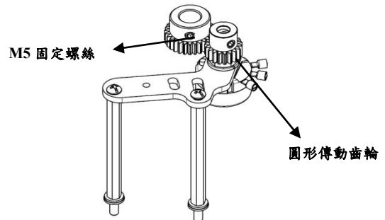
【圓形傳動齒輪】
